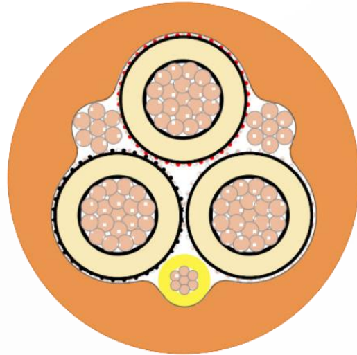
CABLE PORTATIL Y FLEXIBLE TRIPOLAR
